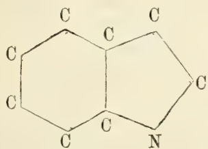
nucleo dell'indolo
